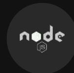
Node.js
